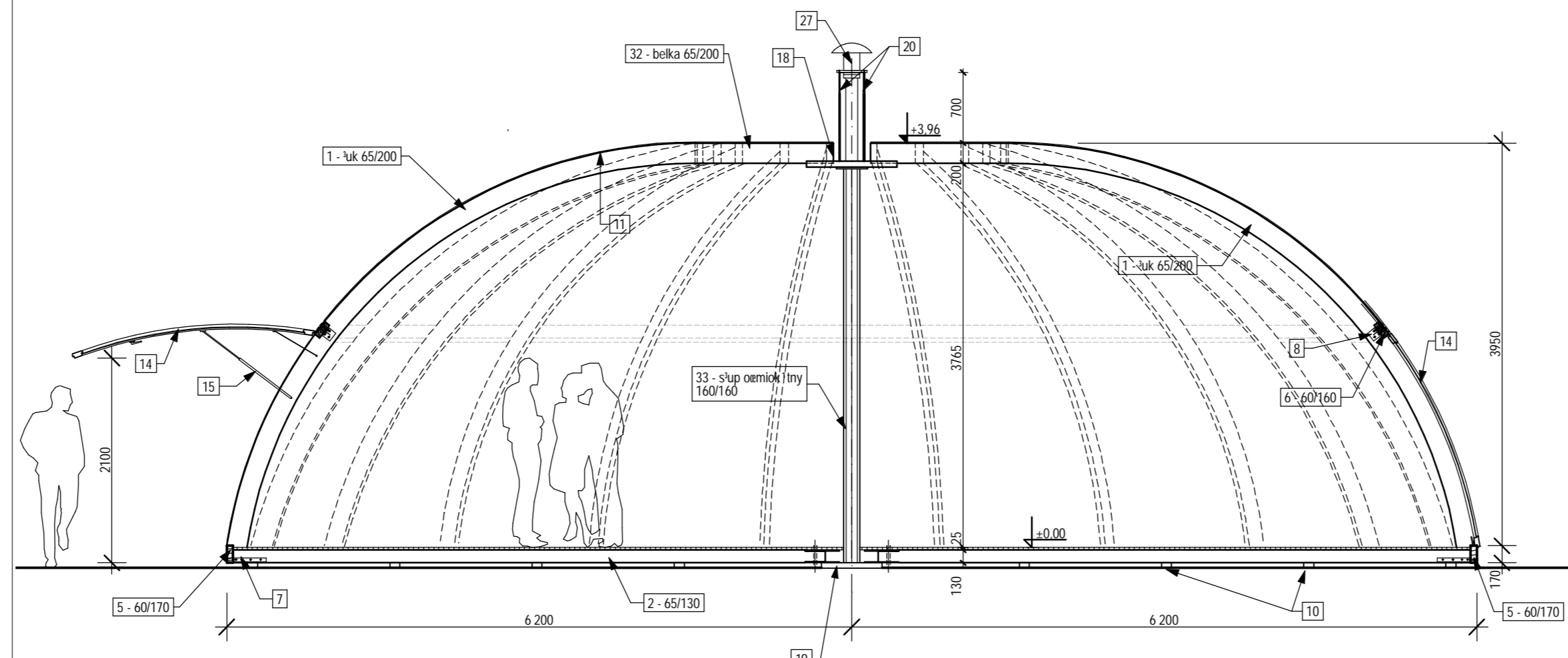
PRZEKRÓJ POPRZECZNY skala 1:50
